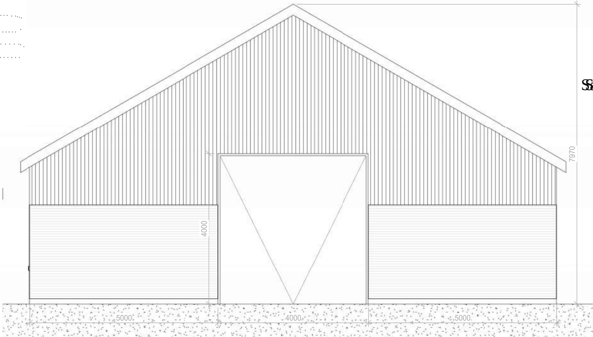
Myndighed - Facade mod vest - Fremtidig | 1 : 100
