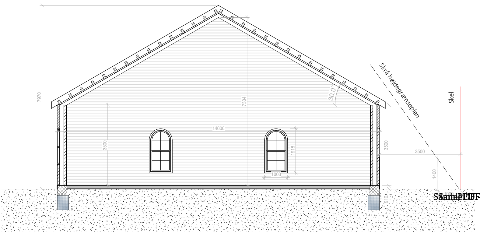
Myndighed - Snit AA - Fremtidig | 1 : 100
