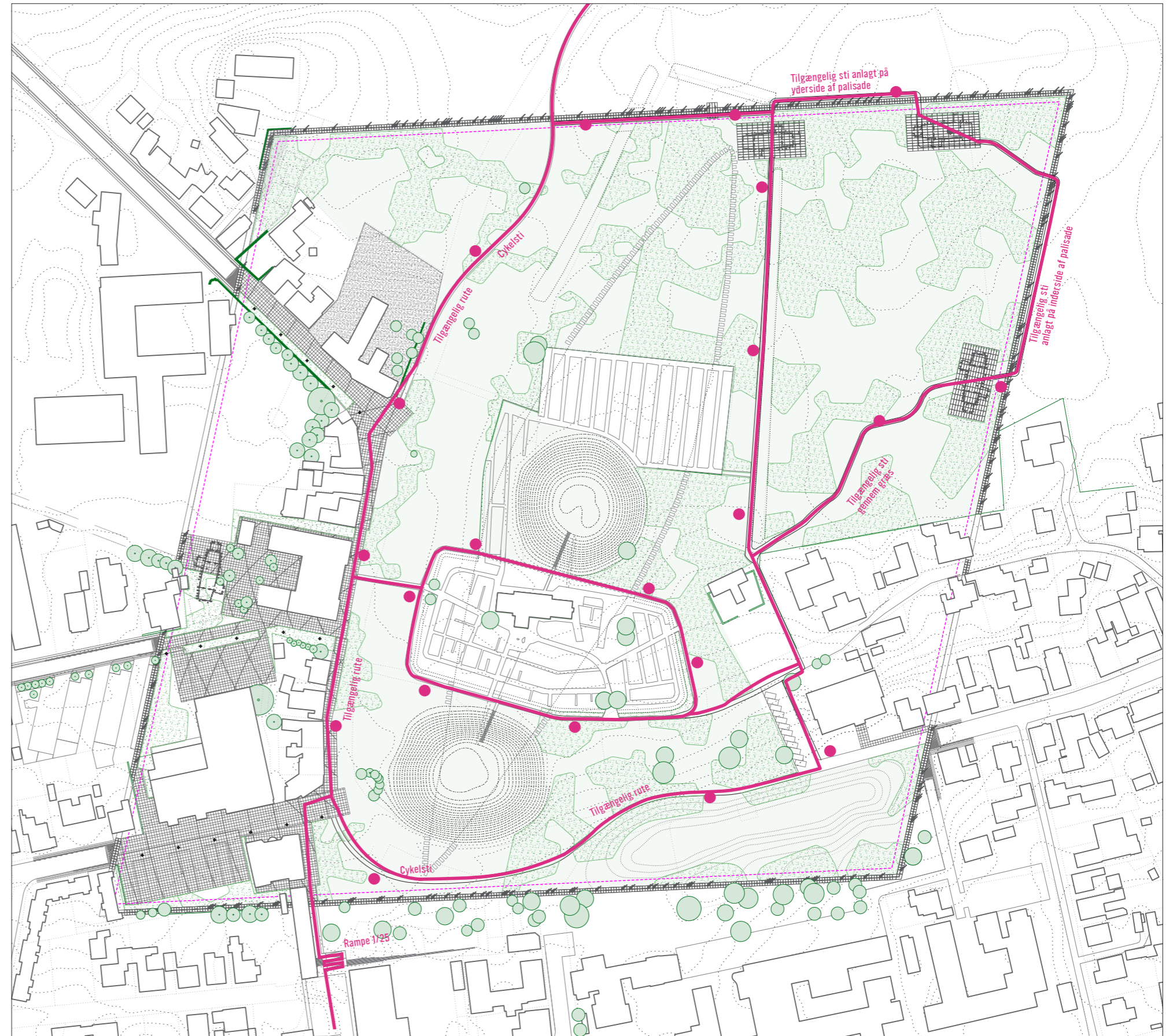
TILGÆNGELIGT STISYSTEM 1:2000
