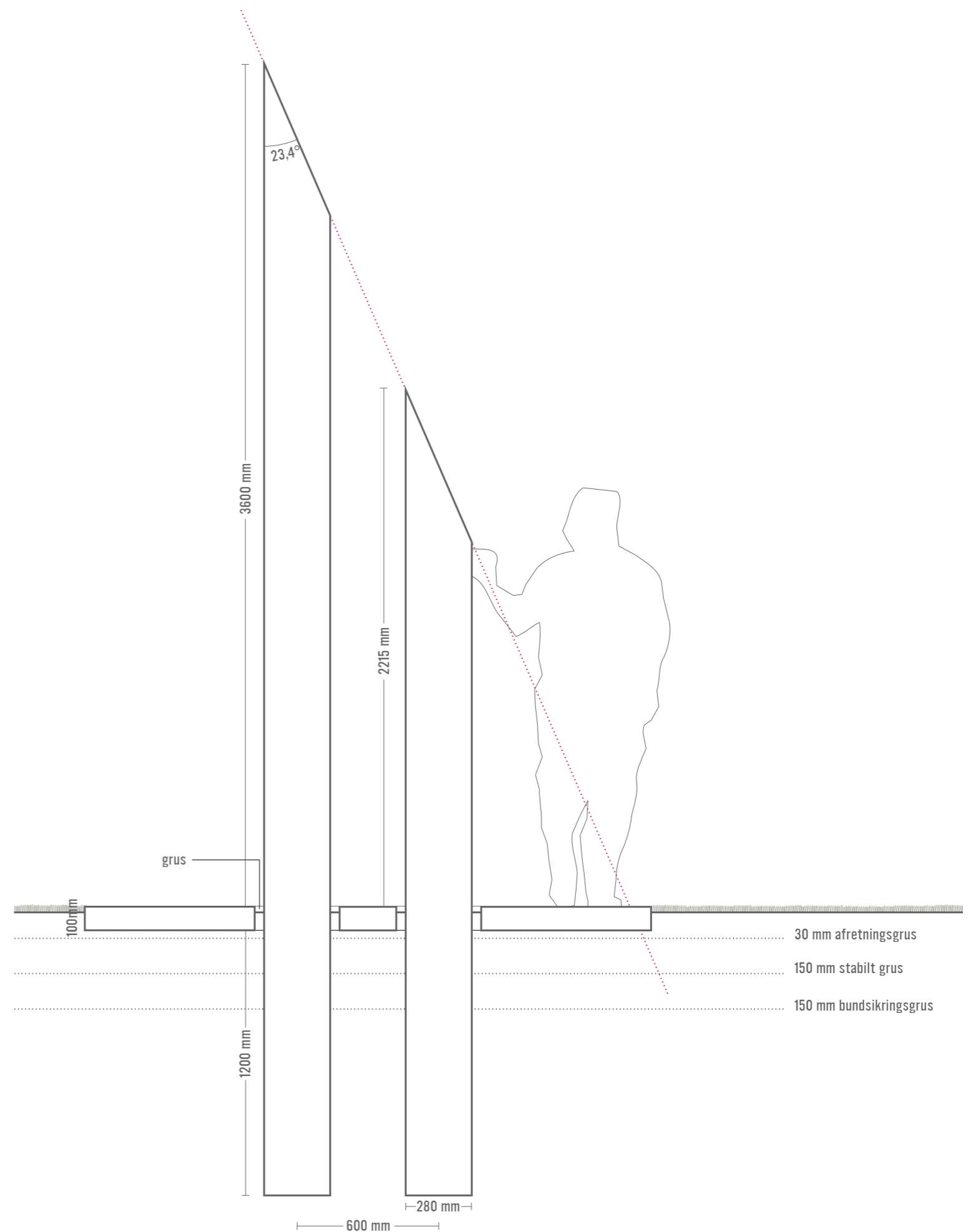
SNIT 1:20
