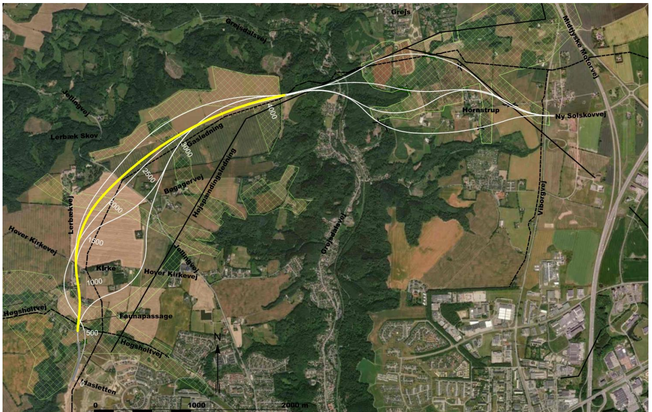
Figur 4-18 Linjeforslag B.
