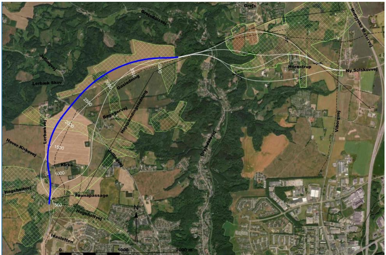
Figur 4-16 Linjeforslag A.
