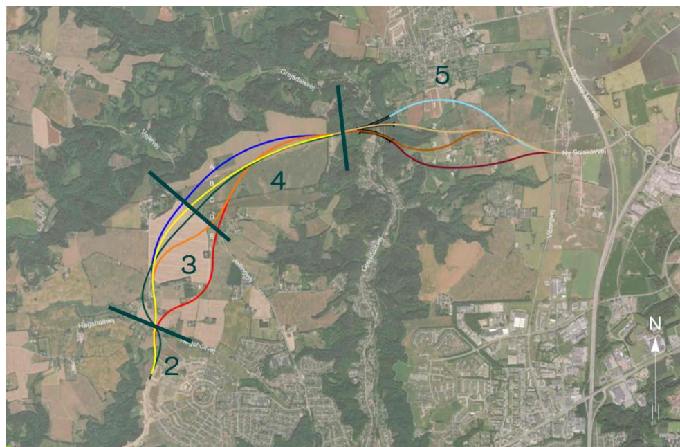
Figur 4-2 Forventet etapeopdeling.
