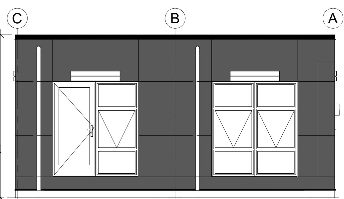
Øst facade 1 : 50
