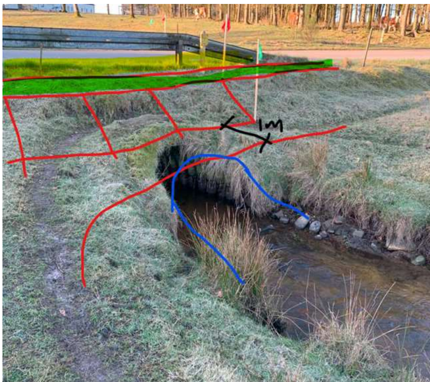
Figur 3 Nuværende forhold med påtegnet skitse. Det røde flag markerer vejudvidelsen, det grønne flag arbejdsområdet. Den blå streg viser fremtidig placering af rørudmunding og røde streger viser terræn.
