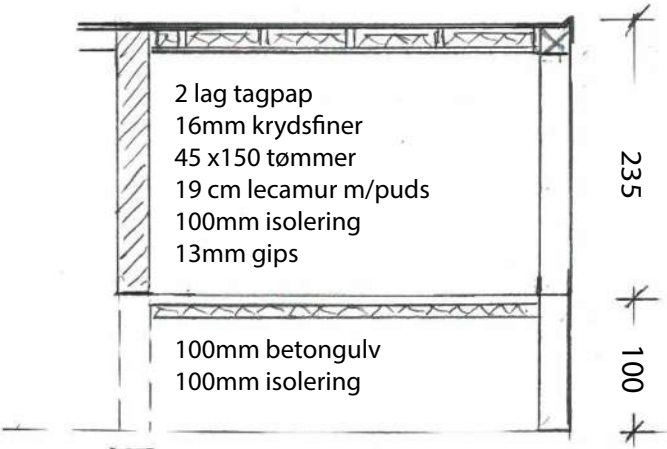
Snit B-B Hobbyrum mål: 1:50
