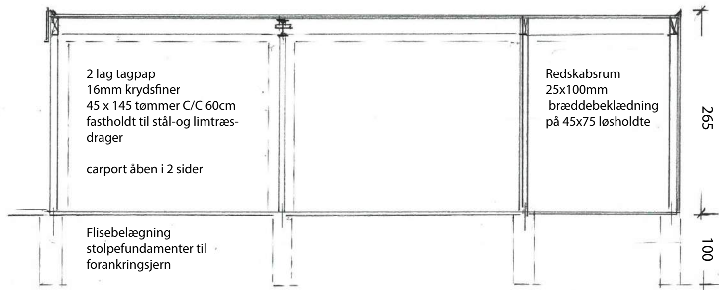
Snit A-A Carport mål 1:50
